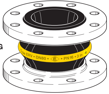
Type ERV-G
